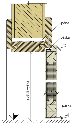
Řez A
