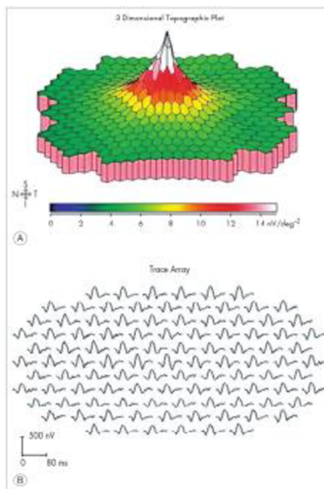
Obr. 13: Normální mfERG [18]
